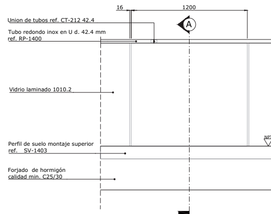
Detalle tramo horizontal tipo Barandilla GlassFit SV-1403 Top F Pasamanos redondo RP-1400 Escala 1:20
