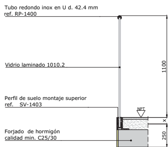
Sección A-A Barandilla GlassFit SV-1403 Top F Pasamanos redondo RP-1400 Escala 1:20
