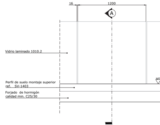
Detalle tramo horizontal tipo Barandilla GlassFit SV-1403 Top F Sin pasamanos Escala 1:20
