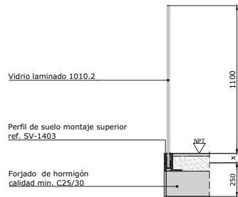
Sección A-A Barandilla GlassFit SV-1403 Top F Sin pasamanos Escala 1:20
